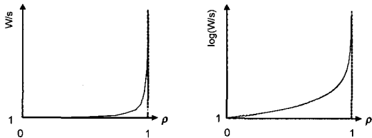
(그림 11) 평균 선회시간에 대한 활용도의 영향
