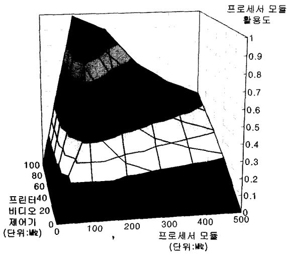
(a) 프로세서 모듈 활용도
