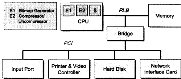
(그림 1) 고속프린터의 구조
