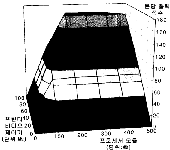
(c) 프린터 비디오 제어기 활용도
