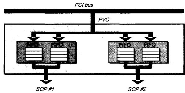
(그림 2) PVC의 구조
