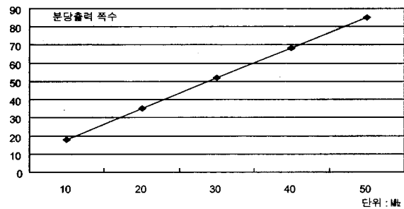
(b) 분당출력 쪽수
