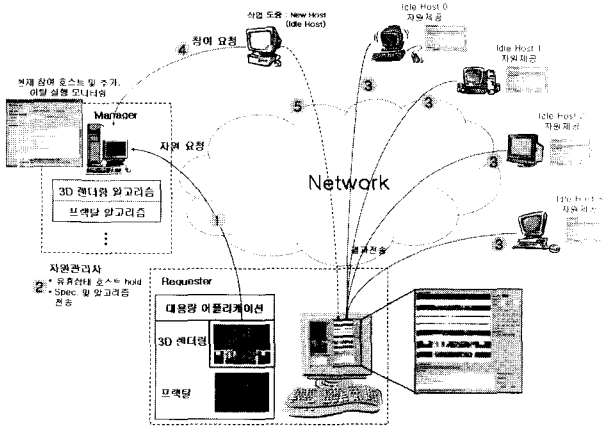
(그림 1) PDP 구성과 제어 흐름
