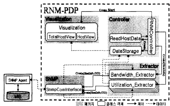
(그림 2) RNM-PDP 구조
