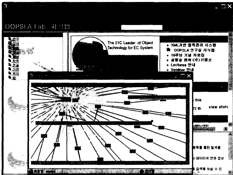
그림 7 K-Box 시스템의 검색유형 - 키워드 검색, 디렉토리 검색, 그래프 네비게이션
