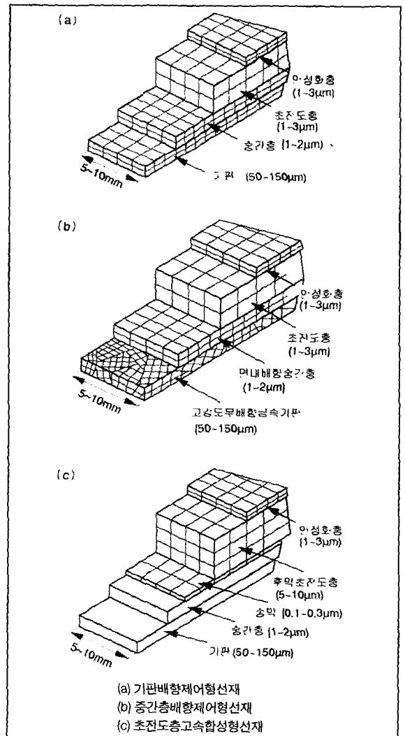
그림 1 차세대 초전도 선재의 구조 모식도
