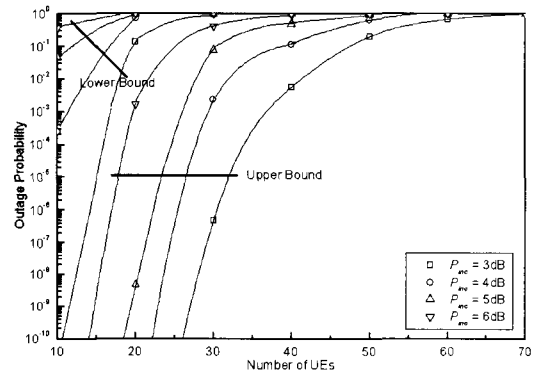
그림 5. TGPL이 4일 때, 단말 수에 따른 에러 확률
