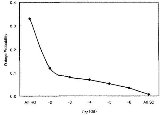
그림 11. 한계치 T_{Tc} 에 따른 에러 확률
