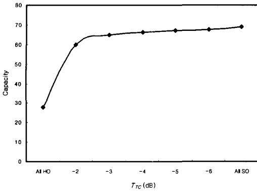
그림 9. 한계치 T_{Tc} 에 따른 용량
