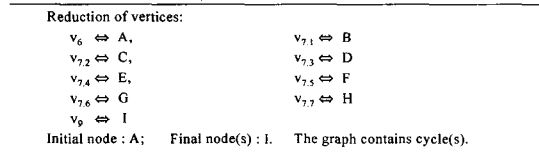
(그림 7) 정점 축소 과정
