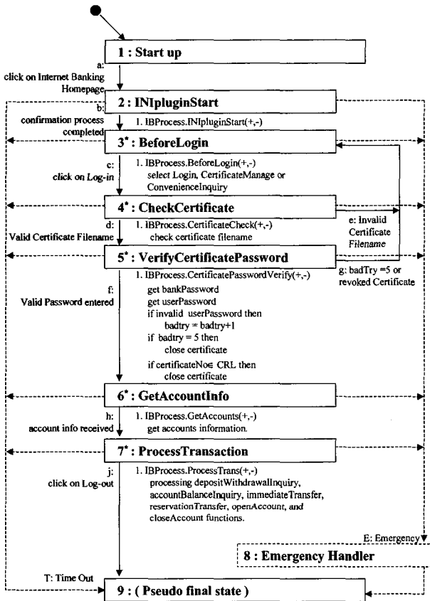
(그림 5) STD : 인터넷뱅킹의 최상위 레벨
