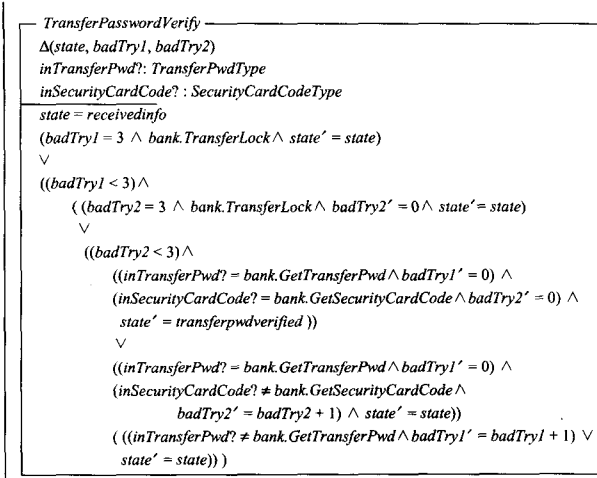
(그림 3) 인터넷뱅킹의 정형적 표현
