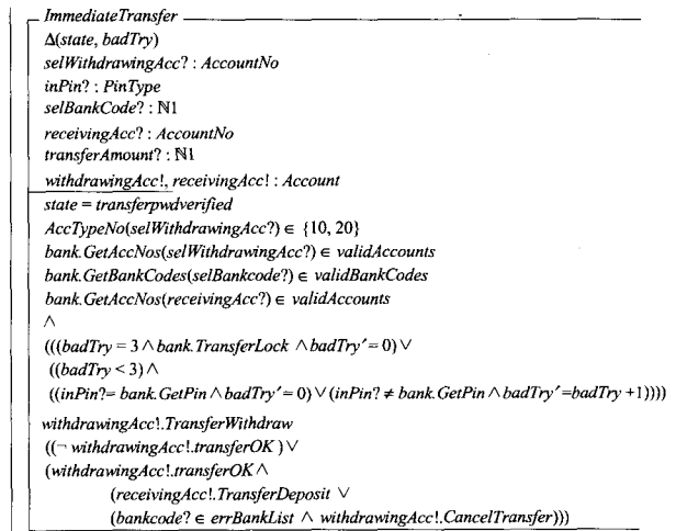
(그림 4) Object-Z 명세 : 즉시 이체
