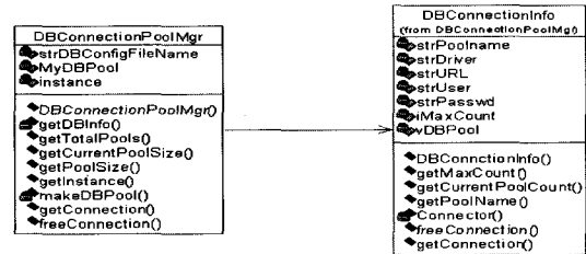
(그림 10) DBConnectionPoolMgr과 DBConnectionInfo 클래스의 다이어그램
