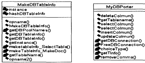
(그림 8) MakeDBTableInfo와 MyDBPorter의 클래스 다이어그램
