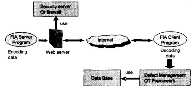
(그림 1) 시스템 구조도
