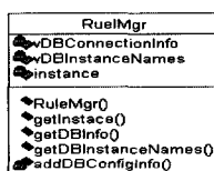
(그림 9) RuelMgr의 클래스 다이어그램
