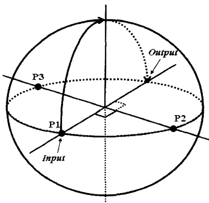
그림 4. 반사형 OCS 셀의 어둠 상태에서의 편광 경로의 Poincaré 구 표현법.
