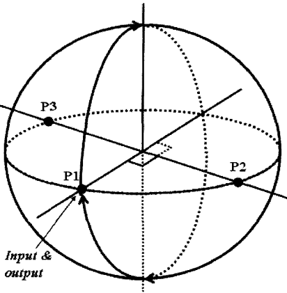
그림 3. 반사형 OCS 셀의 밝음 상태에서의 편광 경로의 Poincaré 구 표현법.
