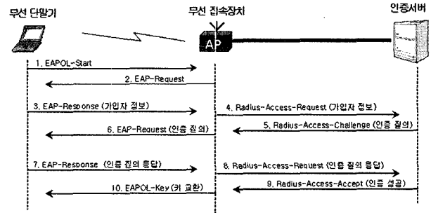
(그림 1) 802.1X 규격에 기반한 무선랜 접속 과정
