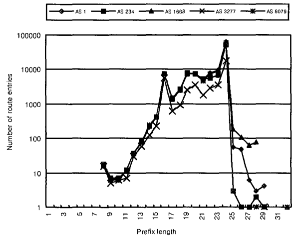
(그림 4) 5개의 AS에 대한 IP 프리픽스 길이의 분포도
