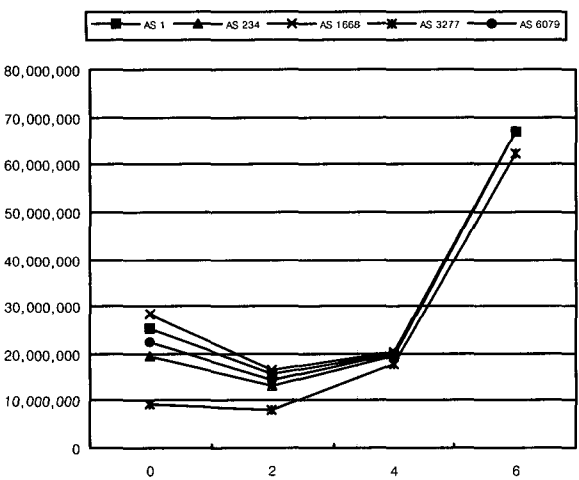
(그림 6) 포워딩 테이블을 저장하는데 요구되는 메모리의 양(Bytes)
