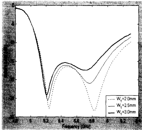
그림 4. W_1 의 길이 변화에 따른 반사계수 특성변화
