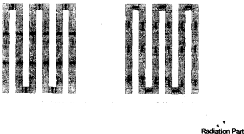
그림 1. 미앤더 선로의 전계 분포와 자계 분포
