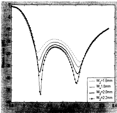
그림 5. W_2 의 변화에 따른 반사계수 특성변화
