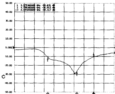
그림 12. 측정된 반사계수
