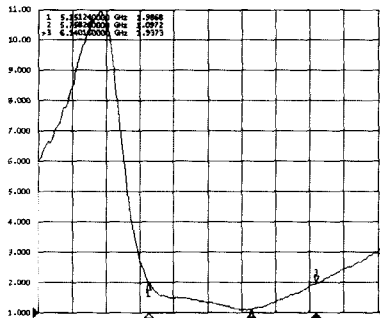
그림 13. VSWR
