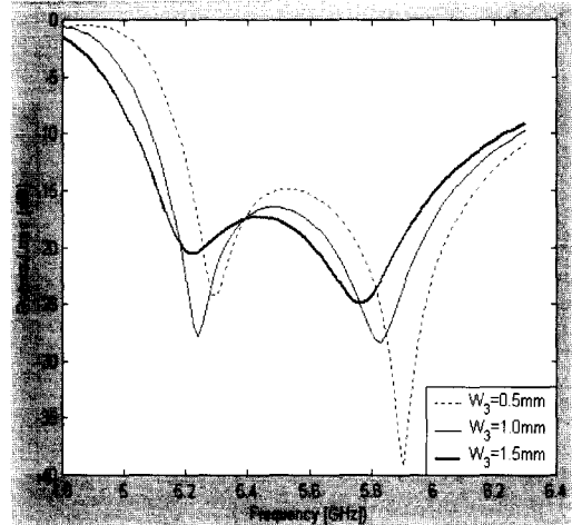
그림 6. W_3 의 변화에 따른 반사계수 특성변화
