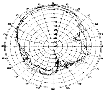
그림 16. Elevation 패턴
