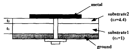
그림 3. 측면도
