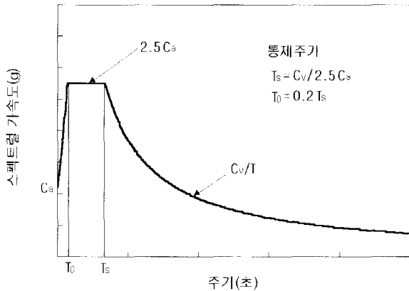
그림 9 내진설계기준연구(II)의 응답스펙트럼
