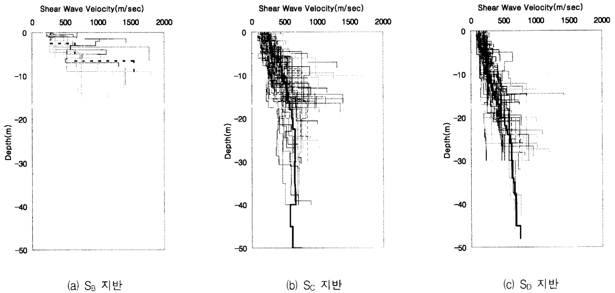
그림 2 지반종류별 깊이에 따른 전단파속도 주상도
