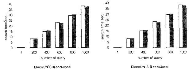
그림 3. 클러스터 시스템에서의 유전자 서열 검색 Fig. 3. Genome sequence analysis at cluster system
