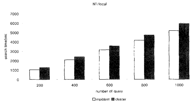
그림 4. mpiBLAST를 사용한 유전자 서열 검색 Fig. 4. Genome sequence analysis using mpiBLAST
