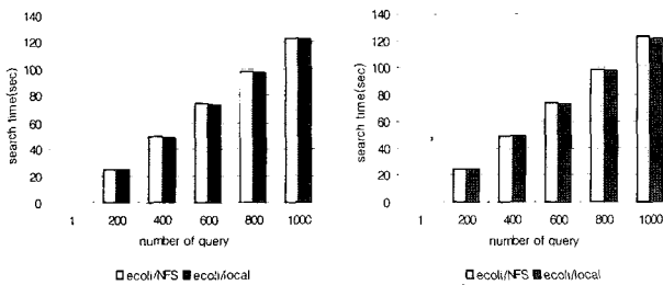
그림 2. 단일 노드에서의 유전자 서열 검색 Fig. 2. Genome sequence analysis at single node
