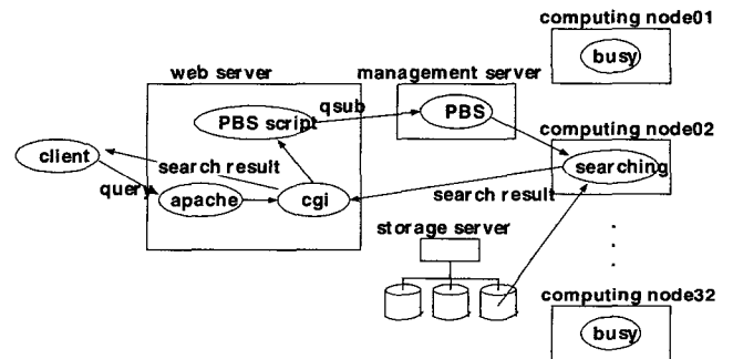
그림 1. 클러스터 시스템 기반 유전자 서열 검색 시스템의 질의 수행 과정
