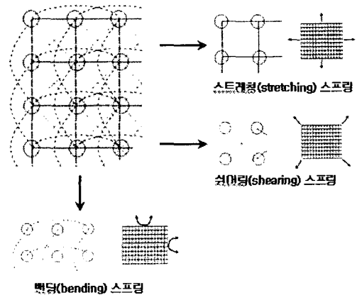
그림 1. 질량-스프링 모델 Fig 1. Mass-spring model
