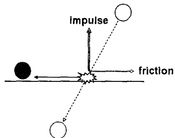
그림 7 충돌 반응 처리 모델 Fig 7. Collision response processing model
