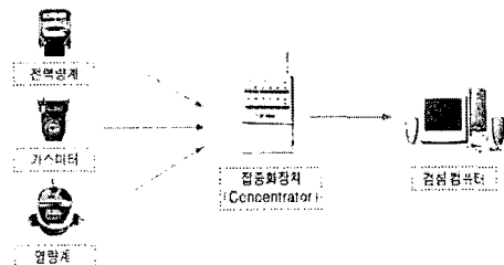
그림 2. 원격검침 시스템 Fig 2. Telemetering system
