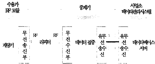
그림 3. 제안한 자동원격검침 시스템 구조도 Fig 3. Structure of proposed AMR system
