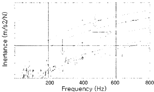
(d) The modification result of body attachment stiffness
