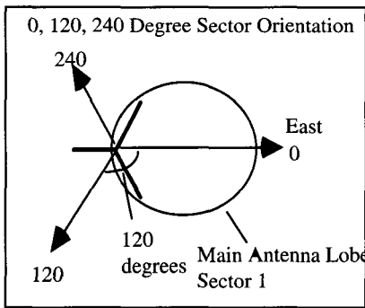
그림 4. 3-섹터 안테나 pattern. Fig. 4. 3-Sector antenna pattern.
