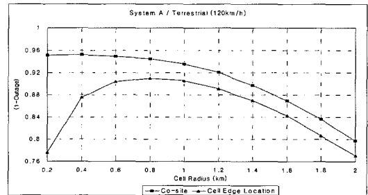
그림 13. Terrestrial (120 km/h) 환경에서 시스템 E의 간섭영향을 받는 시스템 A 셀 반경에 따른 (1-Outage) 특성. Fig. 13. Cell Radius vs. Outage Capacity of System A which is interfering with the System E under terrestrial Terrestrial (120 km/h) environment in case of co-sited and different-sited Gap-filler.
