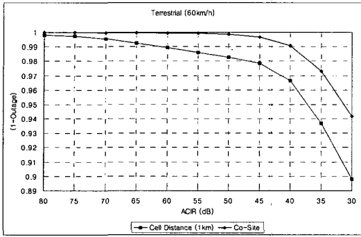
그림 12. 2-Tier 환경에서의 시스템 E 간 거리에 따른 ACIR vs. (1-Outage) 특성. Fig. 12. ACIR vs. Outage Capacity of Sytem E under 2-Tier terrestrial environment in case of co-sited and different-sited Gap-filler.
