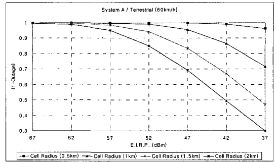
그림 9. 2-Tier 환경에서의 시스템 A의 E.I.R.P. 따른 Outage Capacity. Fig. 9. E.I.R.P. vs. Outage Capacity of System A under 2-Tier environment.
