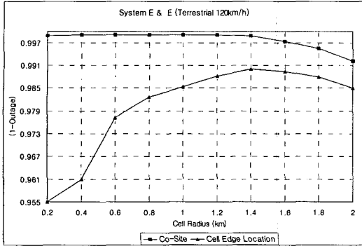
그림 15. Terrestrial (120 km/h) 환경에서 시스템 E의 간섭 영향을 받는 시스템 E 셀 반경에 따른 (1-Outage) 특성. Fig. 15. Cell Radius vs. Outage Capacity of Sytem E which is interfering with the System E under terrestrial Terrestrial (120 km/h) environment in case of co-sited and different-sited Gap-filler.
