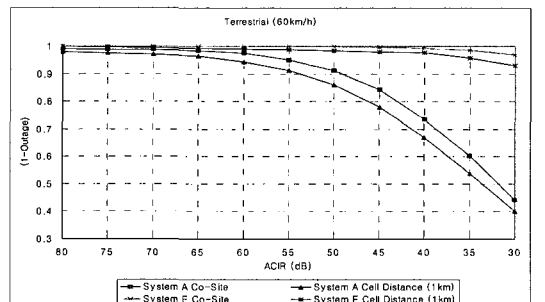
그림 11. 2-Tier 환경에서의 시스템 A와 E 간 거리에 따른 ACIR vs. (1-Outage) 특성. Fig. 11. ACIR vs. Outage Capacity of Sytem A & E under 2-Tier terrestrial environment in case of co-sited and different-sited Gap-filler.
