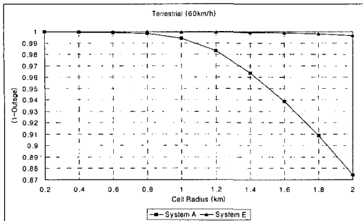
그림 8. 2-Tier 환경에서의 시스템 A와 E의 Cell Radius vs. (1-Outage) 특성. Fig. 8. Cell Radius vs. Outage Capacity of Sytem A & E under 2-Tier environment.
