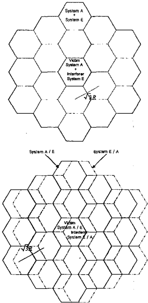
그림 7. 시스템 레벨 간섭 분석 시뮬레이션을 위한 2-Tier 다중 셀 환경. Fig. 7. 2-Tier multi-cell configuration for System-level simulation.
