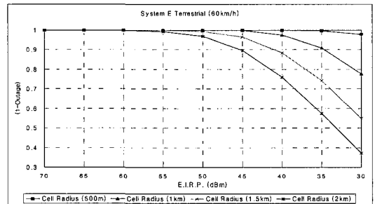
그림 10. 2-Tier 환경에서의 시스템 E의 E.I.R.P.에 따른 Outage Capacity. Fig. 10. E.I.R.P. vs. Outage Capacity of System E under 2-Tier environment.
