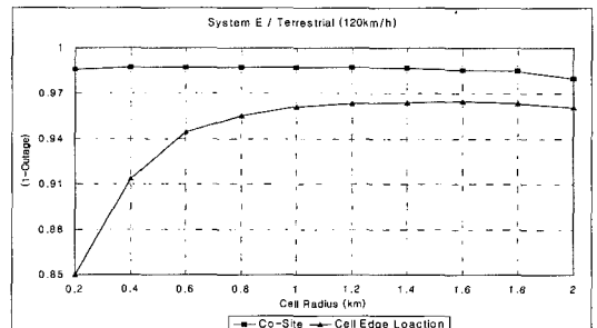
그림 14. Terrestrial (120 km/h) 경우, 시스템 A의 간섭영향을 받는 시스템 E 셀 반경에 따른 (1-Outage) 특성. Fig. 14. Cell Radius vs. Outage Capacity of System E which is interfering with the System A under terrestrial Terrestrial (120 km/h) environment in case of co-sited and different-sited Gap-filler.
