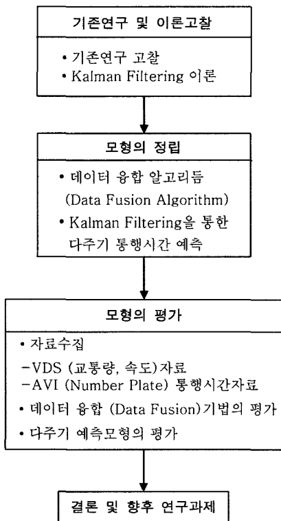
<그림 1> 연구의 수행과정
