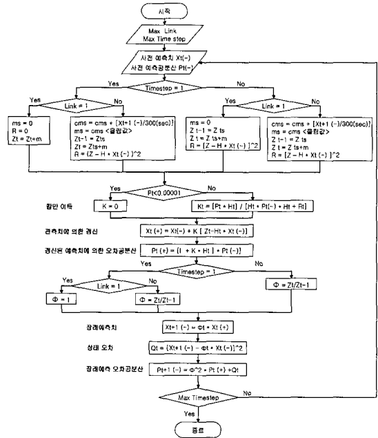
(그림 5) Kalman Filtering을 통한 다주기예측 수행과정도 예측과 동일한 관측방정식이 성립한다(전정규, 2003). Kalman Filtering을 통한 다주기예측의 수행과정은 (그림 5)와 같다.
