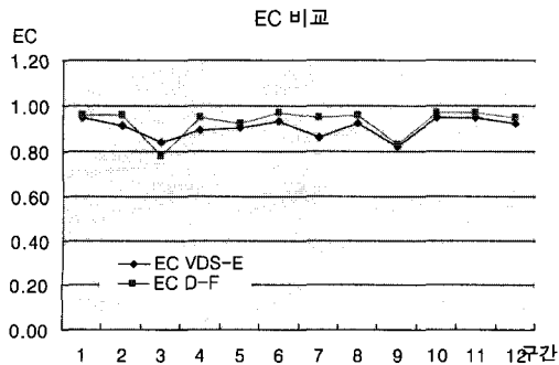
〈그림 10〉 VDS 추정 vs 데이터 융합 EC 비교
