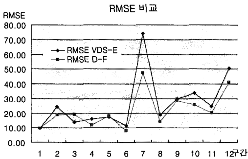
〈그림 9〉 VDS 추정 vs 데이터 융합 RMSE 비교
