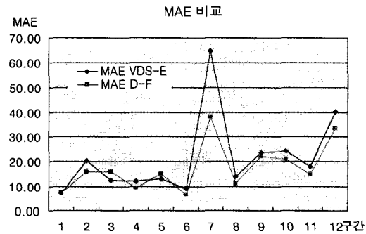
〈그림 8〉 VDS 추정 vs 데이터 융합 MAE 비교
