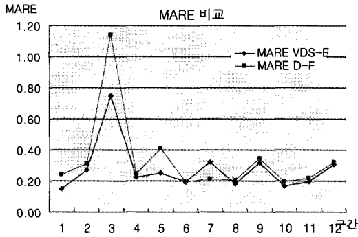
〈그림 7〉 VDS 추정 vs 데이터 융합 MARE 비교
