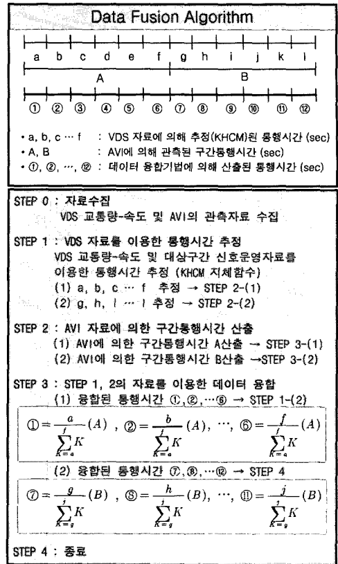
<그림 2> 데이터융합 알고리즘
