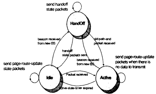
그림 5 핸드오프 상태 머신 캐시 다이어그램 Fig. 5 Handoff State Machine Cache Management State Diagram
