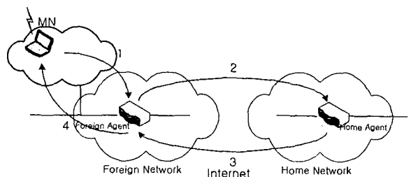
그림 2 에이전트 등록 과정 Fig. 2 Process of Agent Registration
