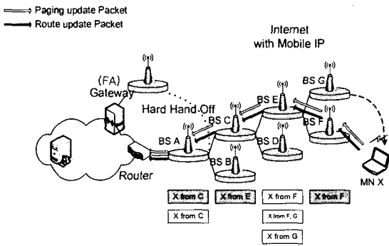
그림 3 페이징 업데이트와 라우트 업데이트 패킷 절차 Fig. 3 Process of Paging-update and Route-update Packet
