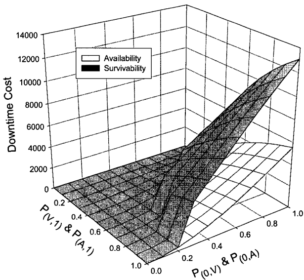
(그림 5) 주-보조서버의 전이확률을 변화에 따른 다운타임 비용 분석
