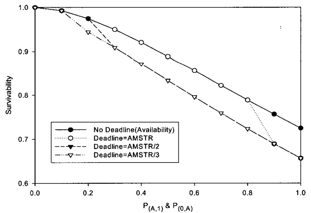
(그림 4) 공격대응능력 및 데드라인 변화에 따른 생존성 분석
