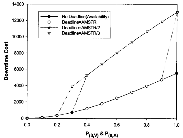
(그림 7) P_{(O,V)} , P_{(O,A)} 및 데드라인 변화에 따른 다운타임 비용 분석
