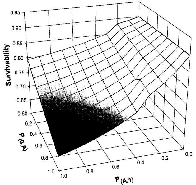
(그림 9) CGI 취약성에 대한 생존성 분석
