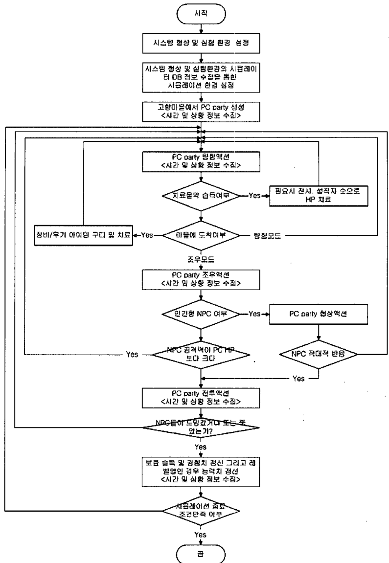
(그림 3) 시뮬레이터 동작 흐름도
