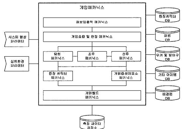
(그림 2) 시뮬레이터 구조
