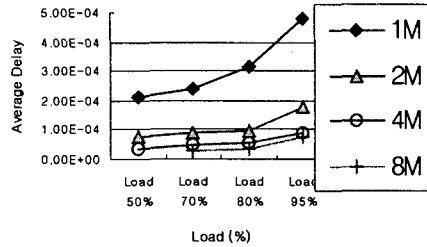
그림 9. 부하량에 따른 평균 지연 Fig. 9 The Average Delay per Load
