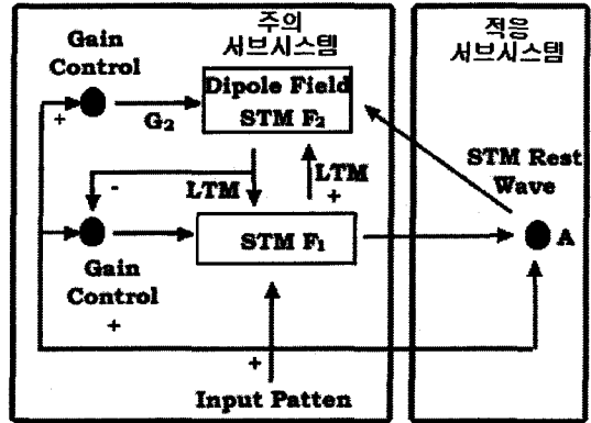
그림 4. ART1 학습 구조 Fig. 4 ART1 learning structure
