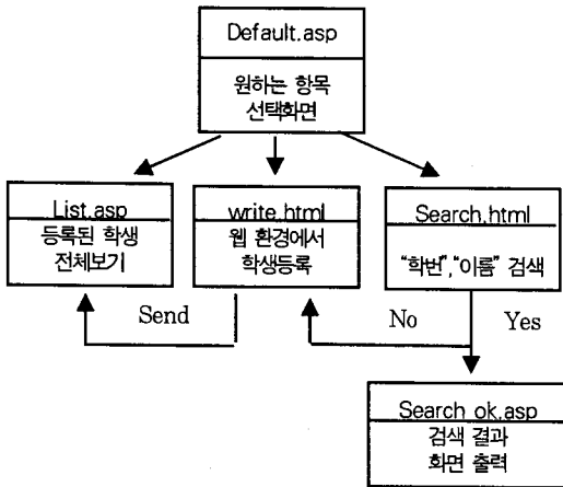
그림 8. 출석부 관리 구성도
