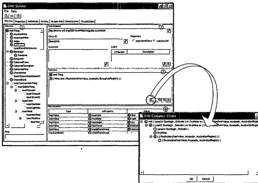
(그림 3) named Class와 complex Class 편집 인터페이스
