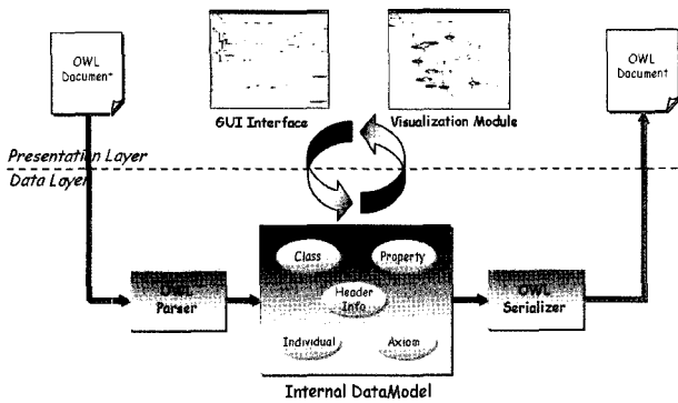
(그림 1) 온톨로지 에디터의 시스템 구조
