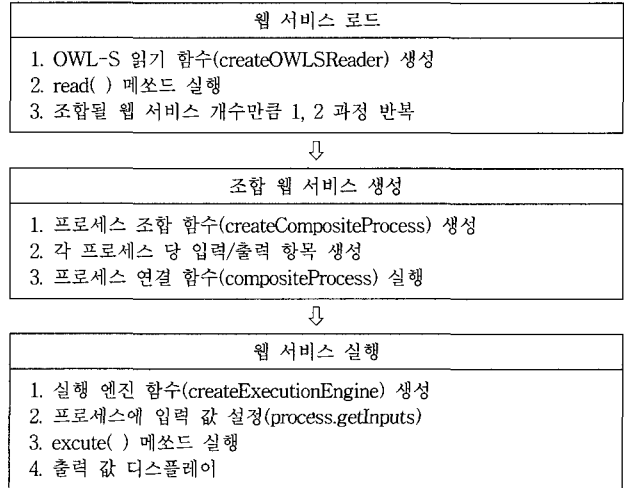
(그림 9) 프로그램 처리 과정
