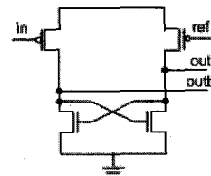
그림 6. 레벨 쉬프터 Fig. 6. Level Shifter.
