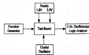
그림 17. 테스트 셋업 Fig. 17. Test Setup.
