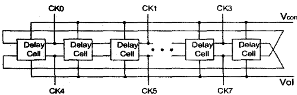
그림 3. 클럭 생성기의 블록도 Fig. 3. The block diagram of Clock Generator.
