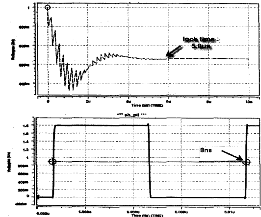
그림 10. PLL의 Locking 시간 및 클럭의 주기모의실험 Fig. 10. Locking time and period of PLL.
