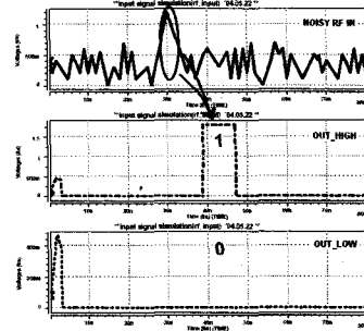
그림 12. 아날로그-디지털 변환기 모의실험 결과 Fig. 12. Simulation result of A/D converter.
