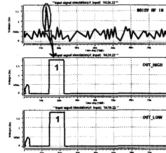
그림 13. 아날로그-디지털 변환기 모의실험 결과 Fig. 13. Simulation result of A/D converter.
