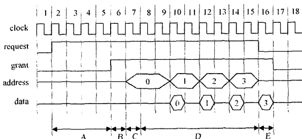
그림 4 트레이스 기반 시뮬레이터의 버스 프로토콜에 따른 4-워드 데이터 전송의 예
