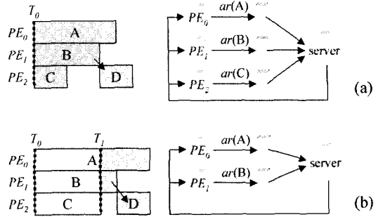
그림 3 (a) 프로세서 PE_0 , PE_1 , PE_2 의 스케줄과 초기 큐잉 모델, (b) T_1 에서 기능 블록 C의 실행이 완료된 이후의 새로운 큐잉 모델
