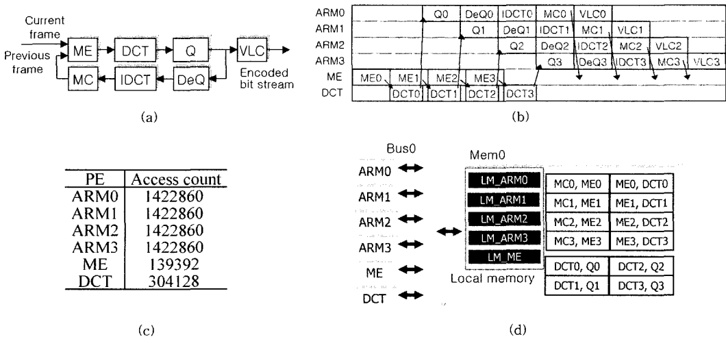
그림 5 (a) H.263 부호기의 명세, (b) 4-채널 DVR의 초기 스케줄, (c) 메모리 트레이스, (d) 단일버스구조 구현
