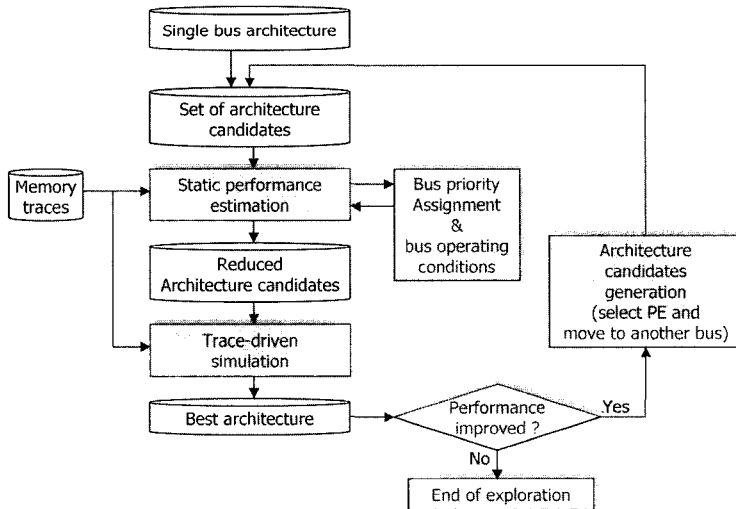
그림 2 제안하는 설계 공간 탐색의 흐름도
