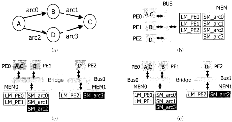
그림 1 (a) 제시된 예제에 대한 블록 다이어그램 표현, (b) 단일버스구조 구현, (c)와 (d) 이중버스구조를 이용한 구현, 각 구현은 공유 메모리 세그먼트인 SM_arc2와 SM_arc3이 각각 다른 버스에 할당되어 있다.
