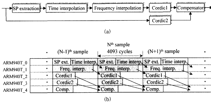
그림 8 (a) OFDM DVB-T 수신기를 위한 이퀄라이저의 명세와 (b) 스케줄
