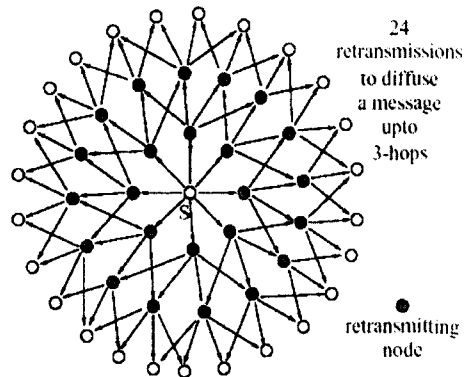
<그림 4> 클러스터링 없이 패킷 전송 <Fig 4> Without clustering of packet transmission
