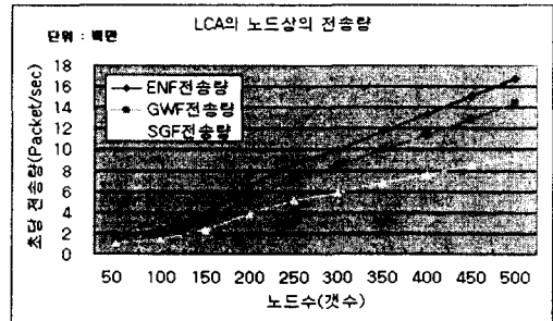
<그림 11> 최저연결 알고리즘 노드상의 전송률 <Fig 11> Transmission rate of LCA
