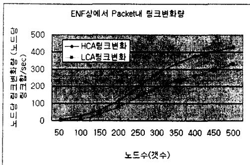
<그림 9> ENF상에서 패킷내 링크 변화량 <Fig 9> Link conversion rate of ENF
