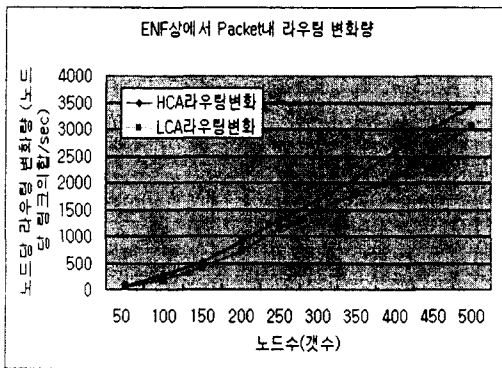
<그림 8> ENF상에서 패킷내 라우팅 변화량 <Fig 8> Conversion rate of ENF
