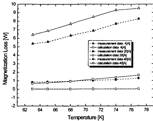
그림 7 측정된 값과 계산 값의 비교 Fig 7 Comparison between measured and calculated AC loss
