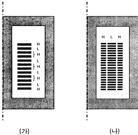
그림 1 교호 / 동심배치 권선 배치 Fig 1 Winding arrangement of each type
