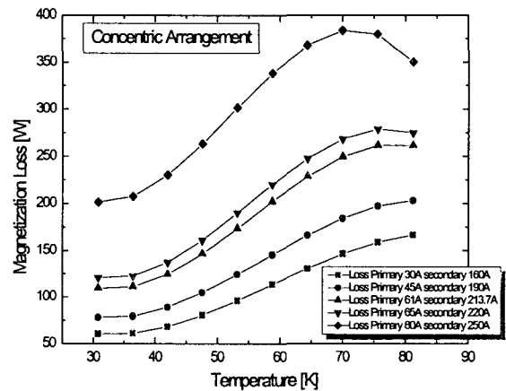
그림 5 동작온도에 따른 자화손실 변화 경향 Fig 5 Tendency of magnetization loss variation according to the operating temperature
