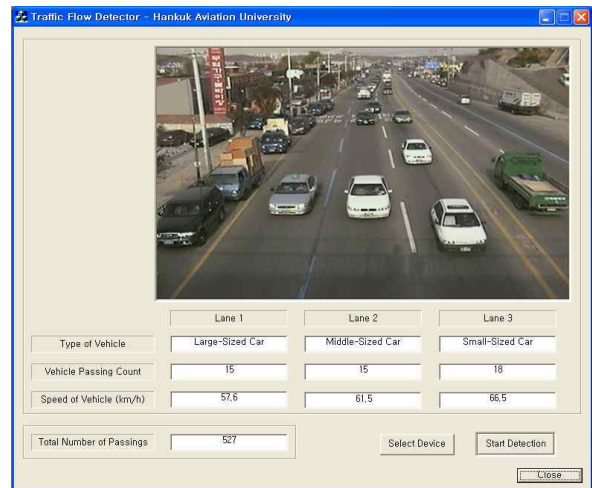
그림 7. 교통량 측정 시스템의 컴퓨터 디스플레이
