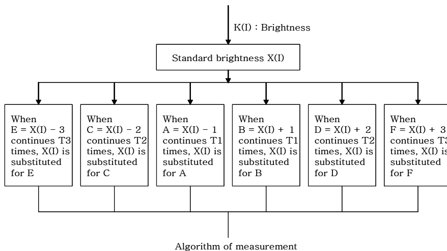
그림 4. 기준 휘도치의 자동조정기법의 흐름도
