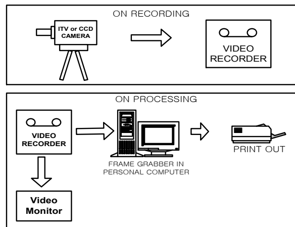
그림 1. 영상처리 시스템의 구성
