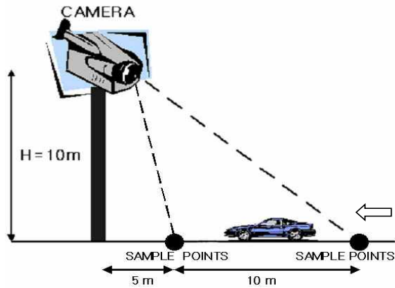
그림 2. 샘플점열과 카메라의 위치 사이의 관계 Fig 2. The relationship between the position of the camera and the sample points
