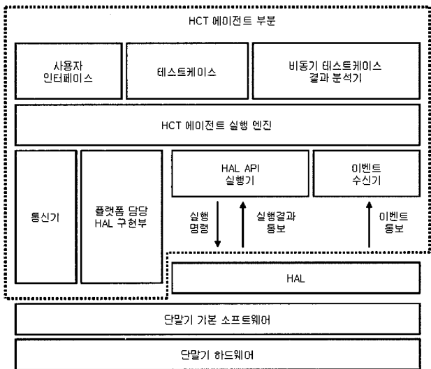
(그림 8) HCT 에이전트 구성도
