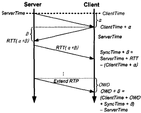
그림 5. 서버/클라이언트 동기화 순서
