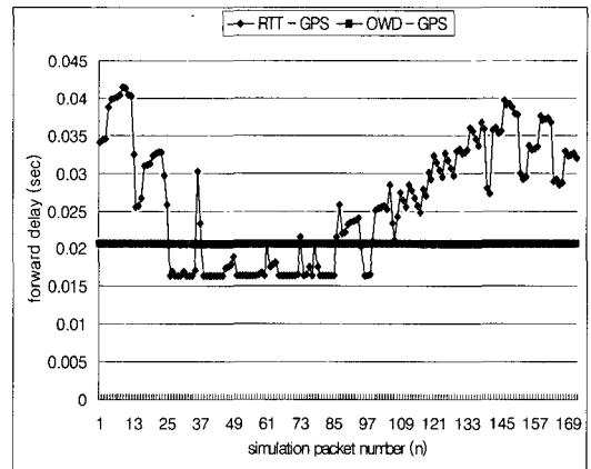
그림 10. 전송 지연
