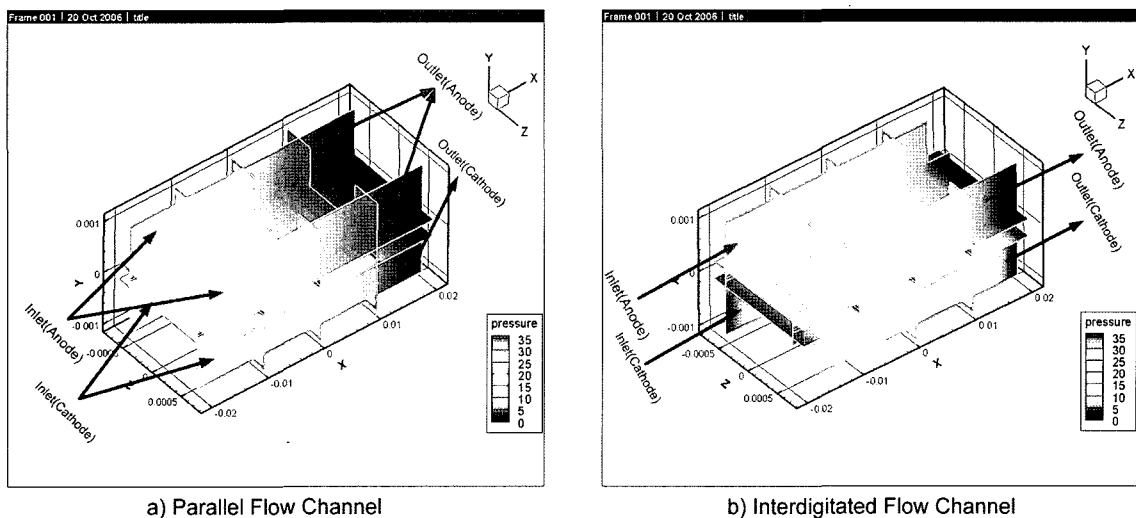
Fig. 5. 채널내의 Pressure drop ( V_{cell}=0.7 V, \Delta P=Pa ).
