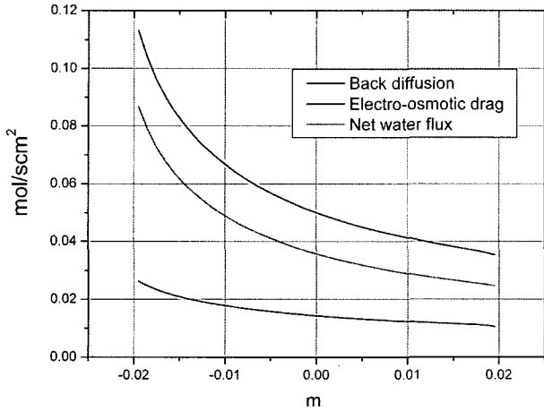
Fig. 8. Parallel유동장에서의 Back diffusion과 Electro-osmotic drag의 길이별 변화 ( V_{cell}=0.7 V).
