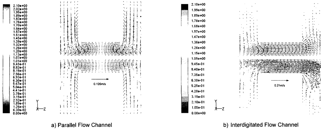
Fig. 4. 유로단면 (Y-Z 면)에서의 속도 분포 ( V_{cell}=0.7 V ).
