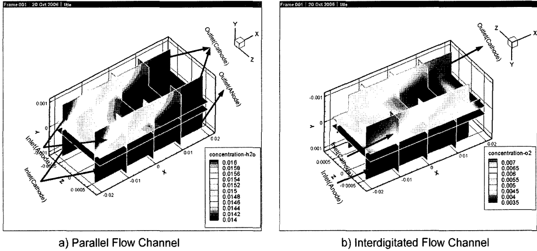
Fig. 6. 공기극에서의 O 2 의 농도분포 ( V_{cell}=0.7\text{ V} ).
