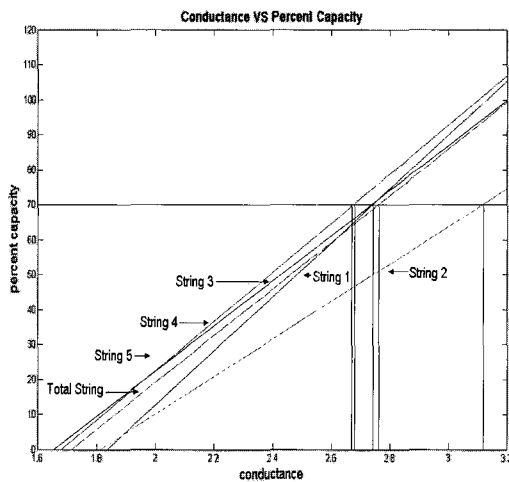
그림 2 각 그룹에 따른 추세선의 차이 Fig. 2 Regression lines from each battery group.
