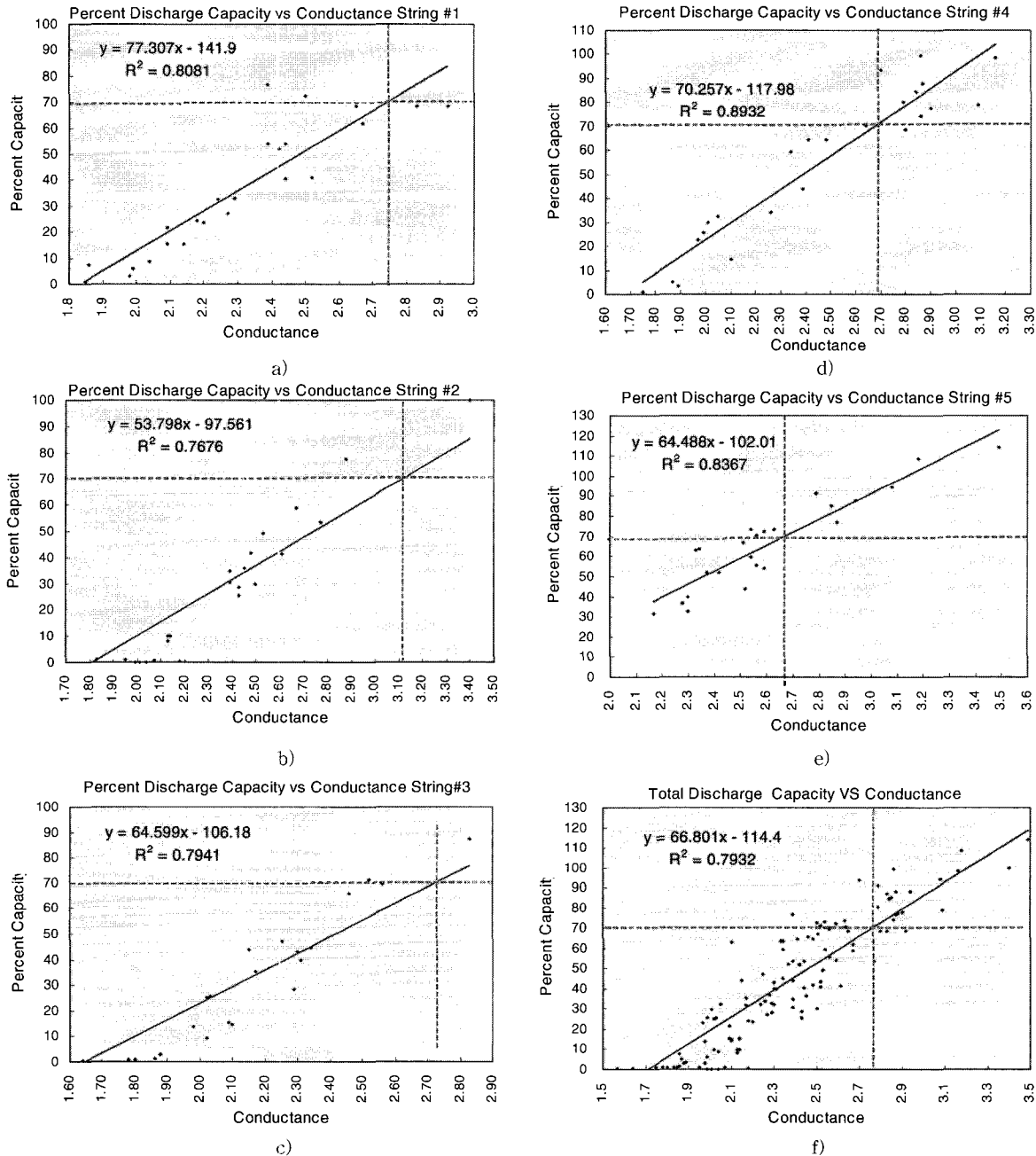
그림 1 5개 납축전지 그룹의 컨덕턴스와 건강상태(SOH)의 상관관계; a) 1그룹, b) 2그룹, c) 3그룹, d) 4그룹, e) 5그룹, f) 총합.
