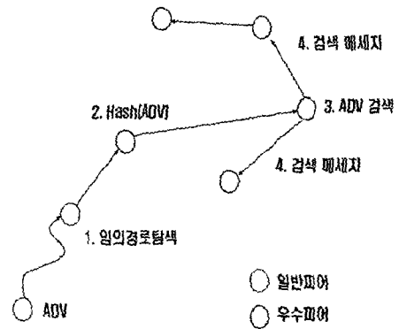
(그림 4) 검색 알고리즘
