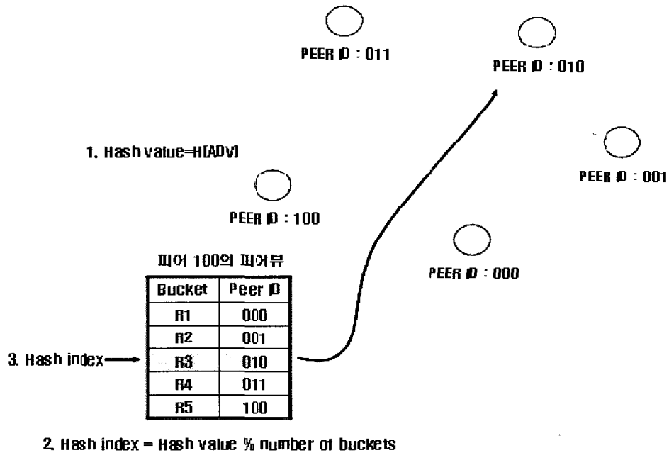
(그림 5) 피어 뷰를 이용한 해싱
