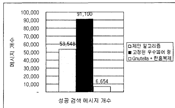
(그림 8) 성공 검색 메시지 개수
