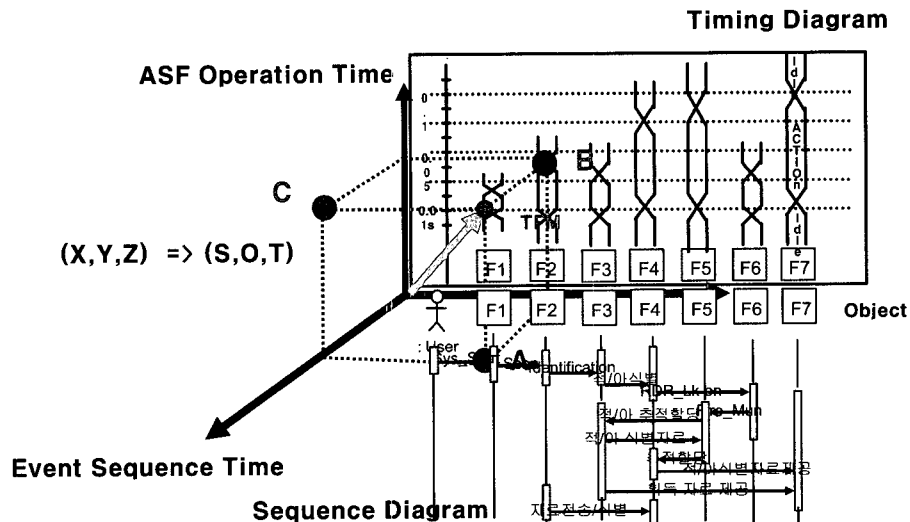
(그림 12) TFM 기반 시스템 테스트 모델 적용사례
