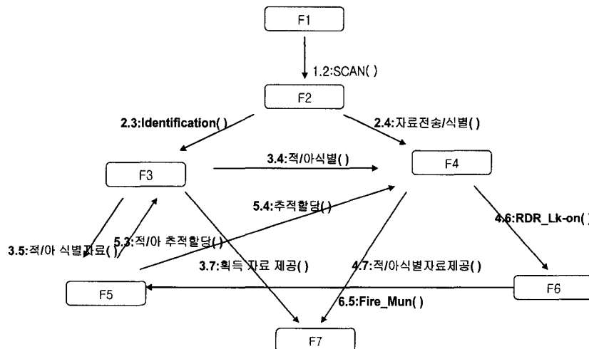
(그림 9) 다기능 미사일 방어시스템의 Collaboration Diagram
