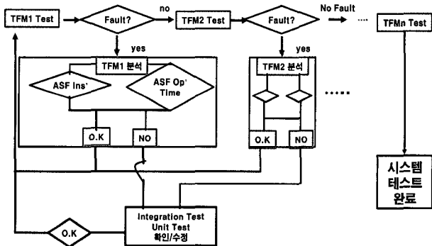
(그림 8) TFM 기반 시스템 테스트 모델 적용방법
