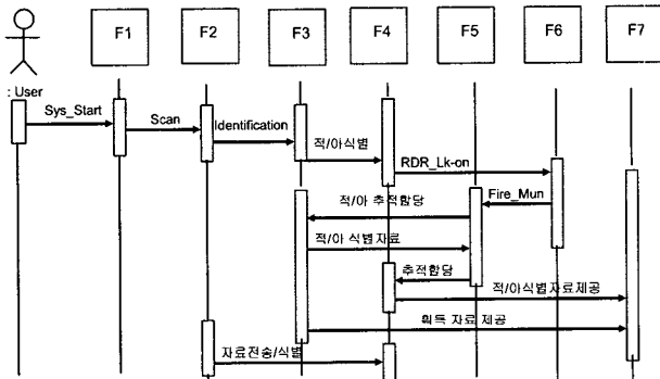
(그림 11) 식별된 Sequence Diagram
