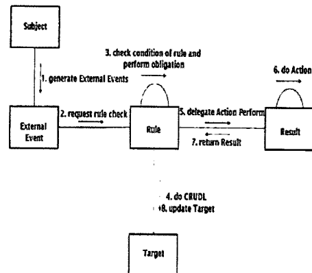
(그림 4) 규칙 기반 분석 패턴의 이벤트 처리 과정
