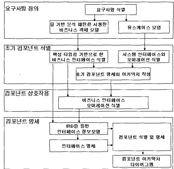
(그림 1) UML Components 개발 프로세스
