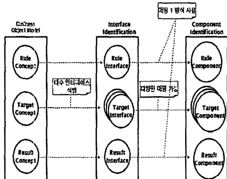
(그림 7) 분석 패턴을 사용한 인터페이스와 컴포넌트간의 매핑
