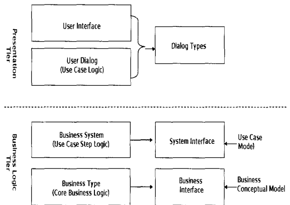
(그림 2) UML Components 어플리케이션 아키텍처
