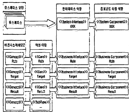
(그림 5) 규칙 기반 분석 패턴을 사용한 인터페이스 및 컴포넌트 식별
