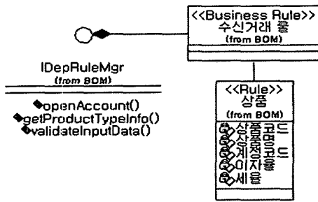
(그림 16) IDepRuleMgr 비즈니스 인터페이스 책임할당 다이어그램
