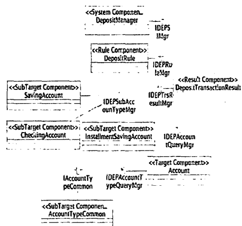
(그림 18) 수신 서브시스템 컴포넌트 아키텍처 다이어그램
