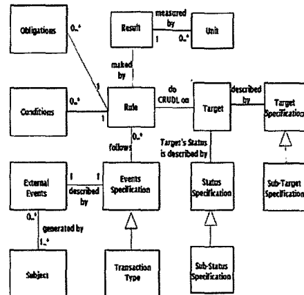
(그림 3) 규칙 기반 분석 패턴 아키텍처 템플릿
