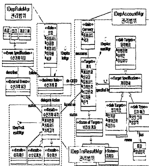
(그림 14) 수신 서브시스템의 핵심 타입과 비즈니스 인터페이스 식별
