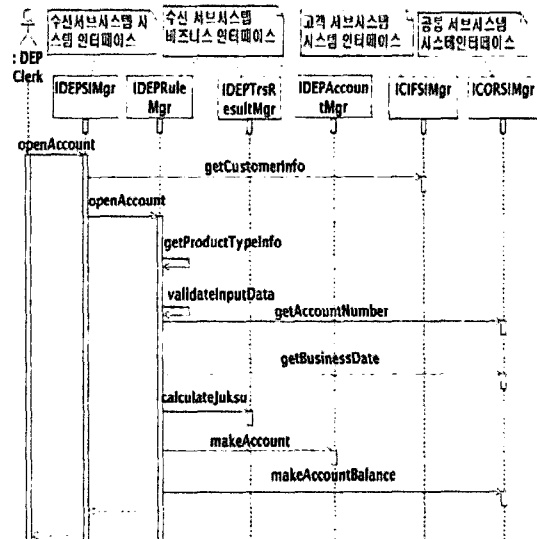
(그림 15) 시퀀스 다이어그램을 통한 계좌 신규 개설 유스케이스 실현 방법
