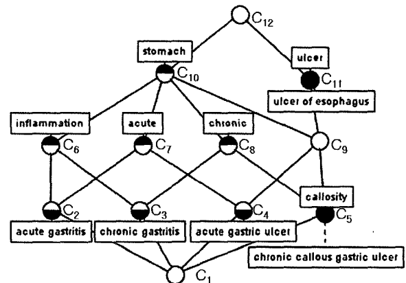
(그림 1) 〈표 1〉의 context에 대한 개념격자
