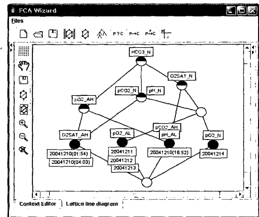
(그림 8) Derived context로부터 개념들을 추출하여 만든 개념격자
