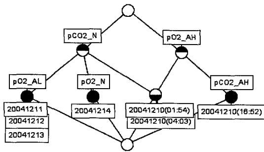
(그림 2) <표 5>에 대한 개념격자
