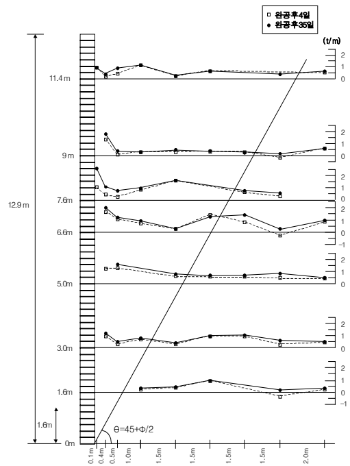
Fig. 9 벽체높이별 보강재의 유발인장력 변화
