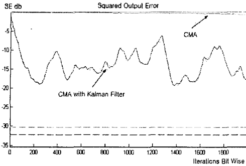
그림 6. 자승오차(BER) 비교 Fig 6. Squared Error Comparison(BER)
