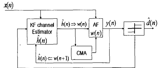
그림 2. 제안한 등화기 구조 Fig. 2 The Proposed Equalizer Structure
