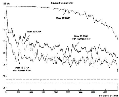
그림 3. 자승오차(BER) 비교 Fig 3. Squared Error Comparison(BER)
