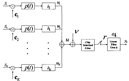
그림 1. DS-CDMA 시스템 Fig. 1 DS-CDMA System
