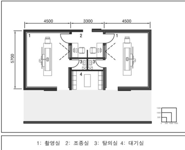
그림 6. 일반촬영유니트 계획안
