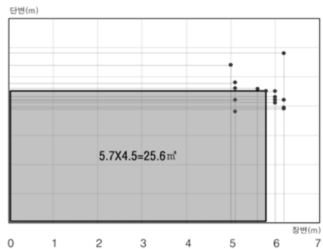
그림 3. 일반촬영실의 면적 (외부 조종실)
