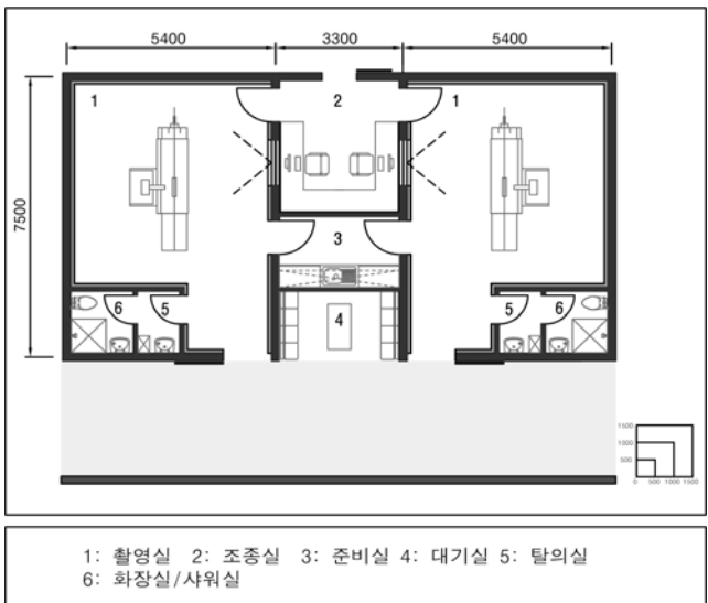
그림 7. 특수촬영유니트 계획안
