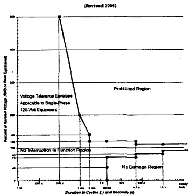
그림 4. ITI 곡선
