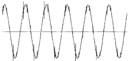
그림 6. Notching 파형
