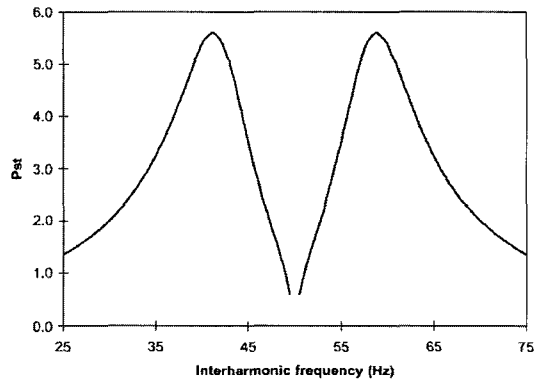
그림 5. Inter-harmonic
