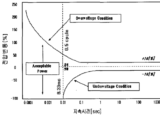
그림 3. CBEMA 곡선.
