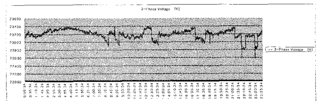
그림 4. 풍력모선전압(2004/10/2)
