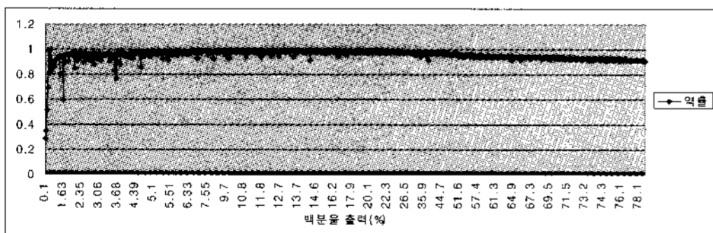
그림 9. 역률(2004/10/1)
