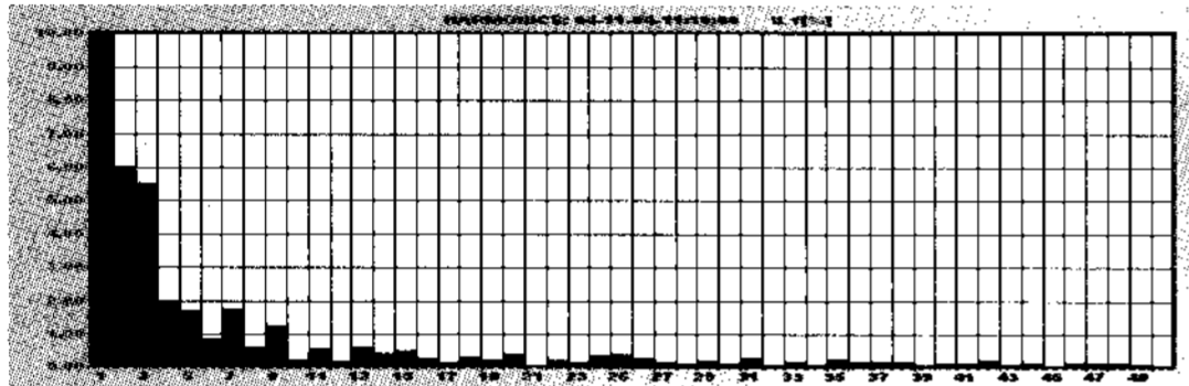
그림 7. 전류고조파(2004/11/4 11:10)
