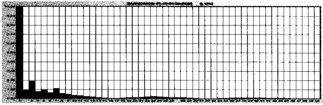
그림 5. 전류고조파(2004/10/1 00:00)
