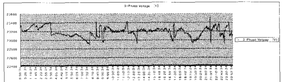
그림 2. 풍력모선전압(2004/10/1)
