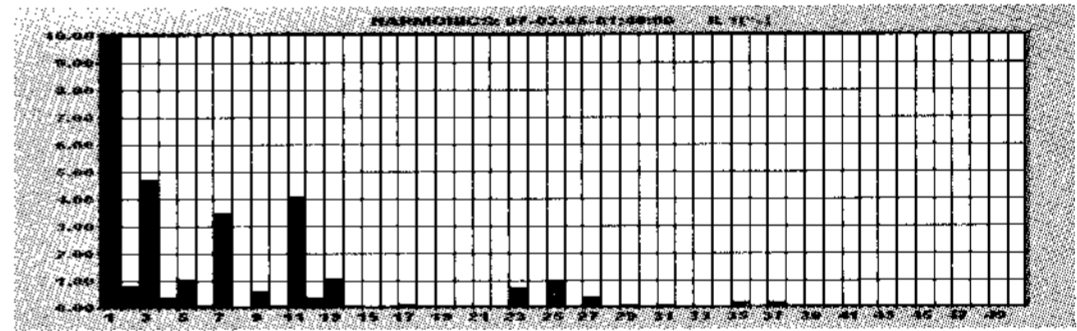
그림 14. 전류고조파(2005/03/07)
