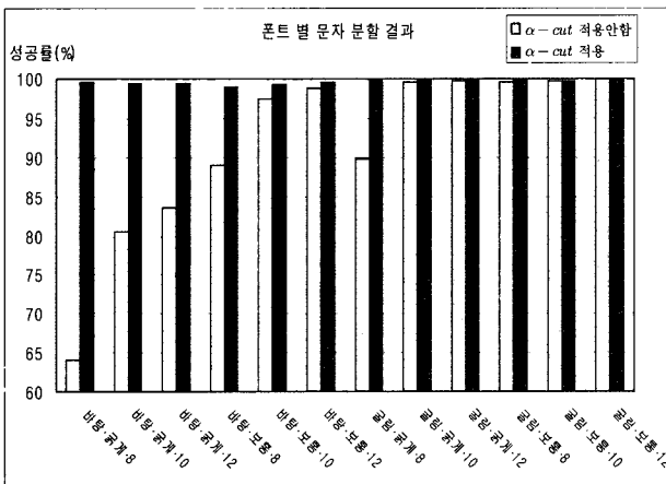
(그림 9) \alpha-cut 적용 여부에 따른 문자 분할 성공률 비교
