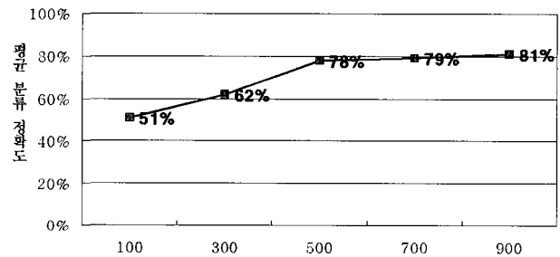
(그림 4) 학습 데이터 양에 따른 분류 정확도 변화
