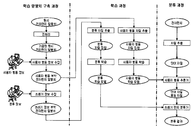
(그림 1) 제안된 쓰레기 편지 여과 시스템의 구조
