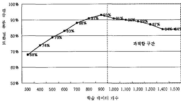
(그림 5) 과적합 현상을 관찰을 통한 학습 데이터의 최적 크기
