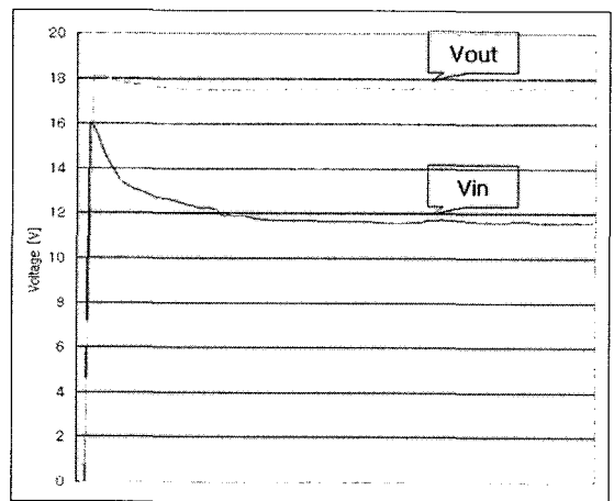
그림 11. 퍼지제어기에 의한 전압 그래프
