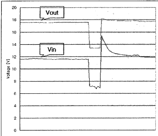
그림 12. 일사량 변화 시 전압 그래프
