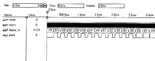
그림 8. 입력에 따른 제어기 시뮬레이션
