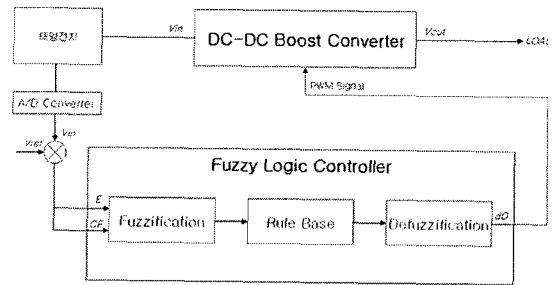
그림 2. 퍼지제어기 구성도
