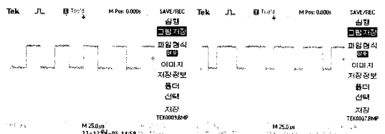
그림 10. 시비율 0.5(좌), 0.7(우)일 때 PWM 출력
