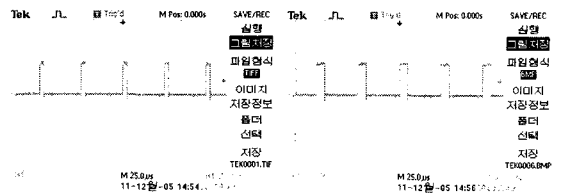
그림 9. 시비율 0.1(좌), 0.2(우)일 때 PWM 출력
