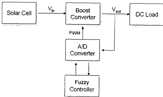
그림 1. 태양광발전시스템의 구성도
