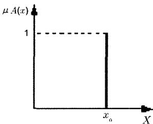
그림 3. 퍼지 싱글톤
