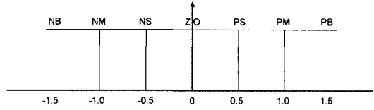
그림 4. 입력변수 CE의 소속 함수
