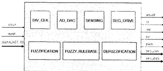
그림 7. 퍼지제어기의 블록도
