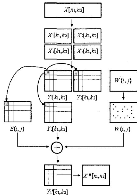
그림 2. 워터마크 삽입 순서도 Fig 2. Watermark Insertion Diagram
