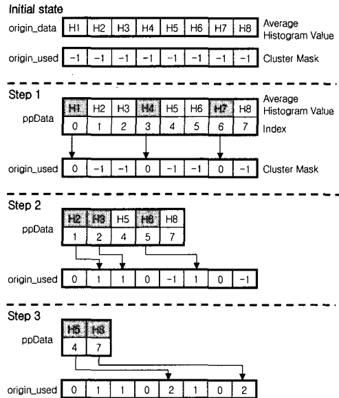
그림 3. 새로운 샷 병합 과정 Fig 3. New Shot Merging Process
