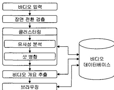
그림 1. 시스템 구조 Fig 1. System Architecture
