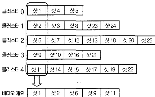
그림 6. 첫 번째 샷을 이용한 비디오 개요의 예 Fig 6. Example of Video Abstracting Using First Shot
