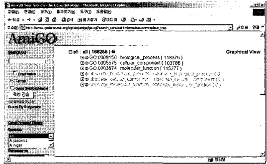
그림 3 AmiGO
