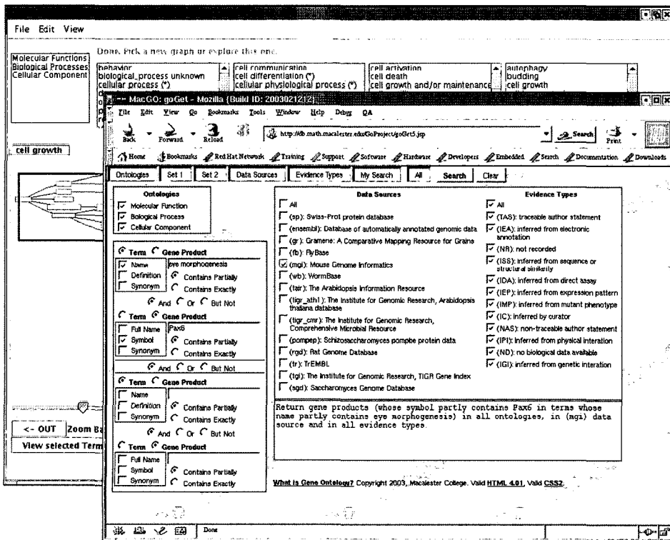
그림 4 GOView & GOGet
