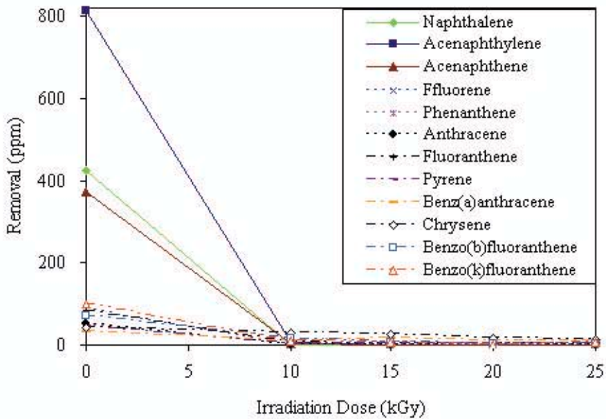
하수슬러지에 포함되어 있는 다양한 종류의 환경위해 화학물질들이 전자선 조사에 의해 제거되는 결과
